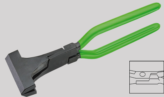
Falzzange gerade, Gewerbe eingelegt, tauchisolierte Griffe
