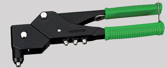
FREUND-Winkelnietzange Kopf 360° drehbar. Jeder Winkel erreichbar, Industriequali- tät, mit vier Mundstückgrößen FREUND-toggle joint hand riveter head 360° turnable, each corner can be reached, industrial quality, with 4 sizes of nose pieces
