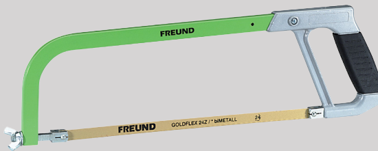
Metallsägebogen, Pistolengriff schwerer Bogen aus Vierkantrohr, 18 x 10 x 1.35mm, Kreuz- schlitzaufnahme, pulverbeschichtet Hacksaw frame professional hack saw frame (for 12" blades), heavy rectan- gulat tube 18 x 10 x 1.35mm, square fittings, durable epoxy finish, bi-component plastic/aluminium pistol-handle
